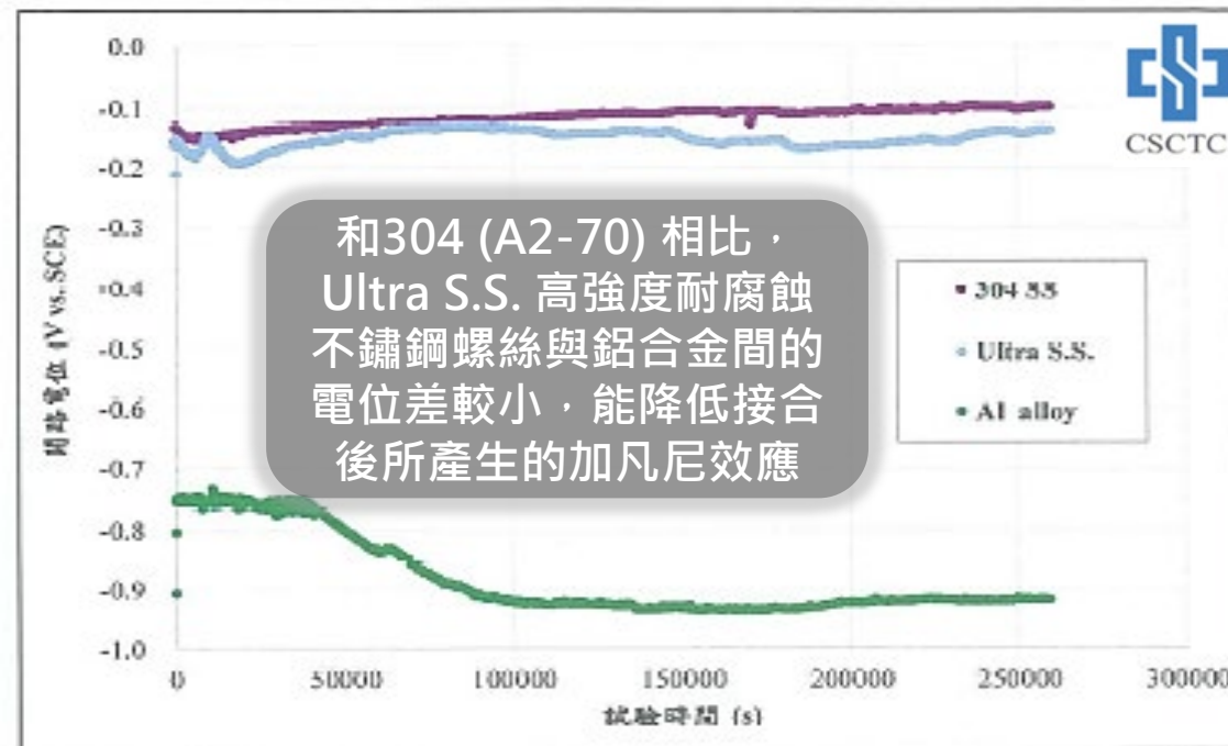
圖 2 試樣於常溫 5 wt.% NaCl 溶液(pH 4.5)中之開路電位曲線
