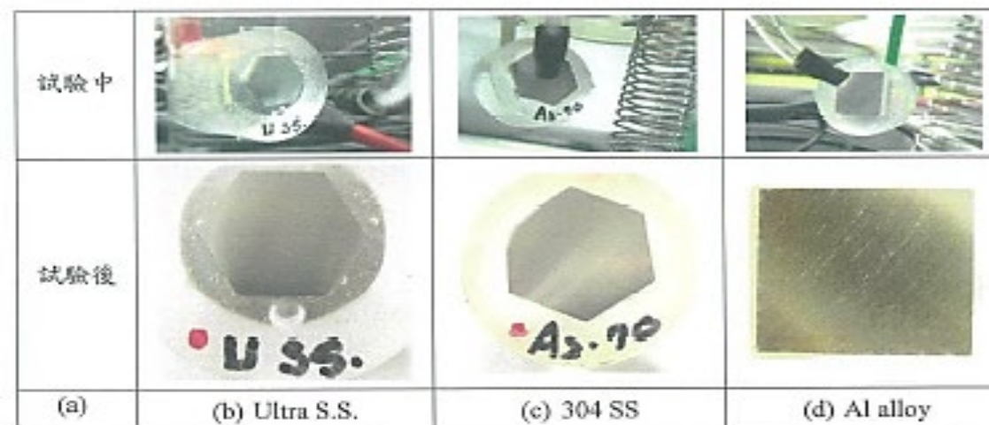
圖 3 試樣在 OCP 試驗中及試驗後之外觀照片
